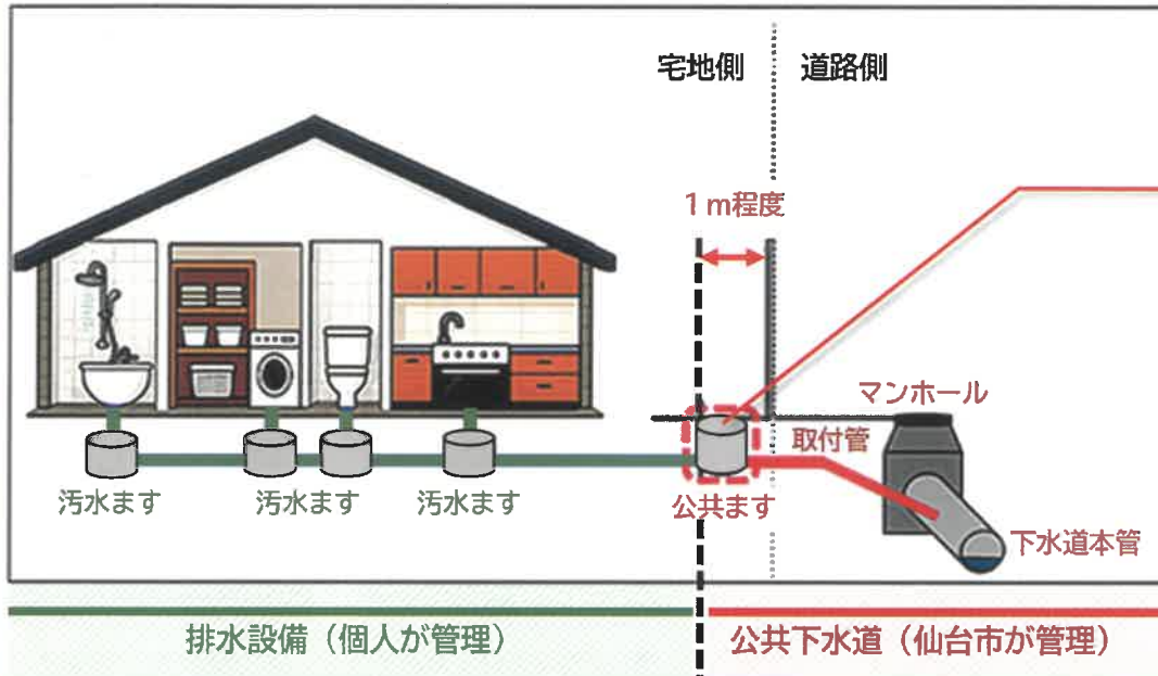
公共ます(汚水)の例
